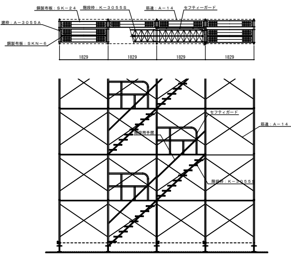
階段 詳細図 1/50
