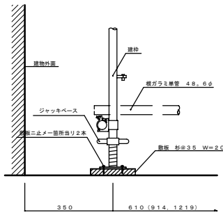
足元部分詳細 1/10
