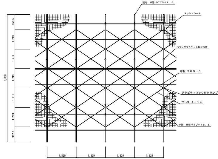
ア-ア断面詳細図 1/50
