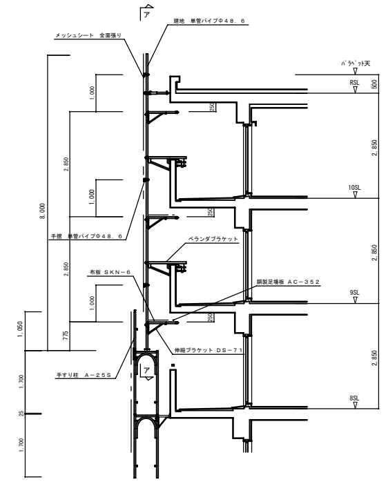
断面詳細図 1/50
