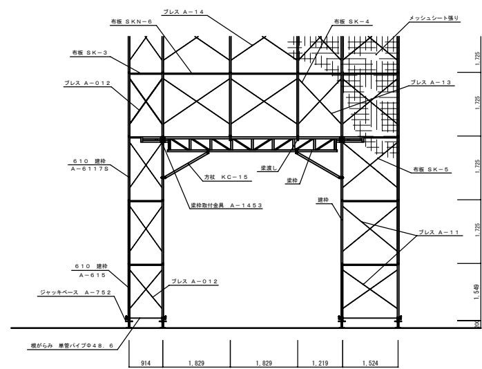
梁枠詳細図 1/50
