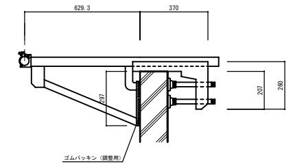
ベランダブラケット取付詳細図 1/10
