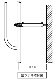
壁ツナギ取付図
