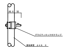
筋交取付部分詳細図 1/5
