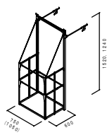
レインボーハンガー (HR-075) 詳細図
