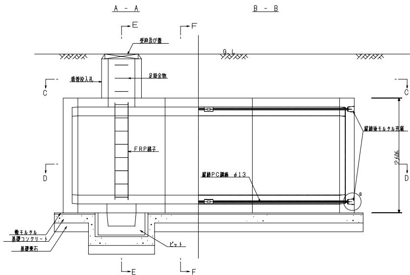
側面図
