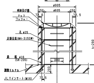
喉管投入孔 S=1/20 断面図
