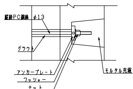
a部詳細図 S=1/6
