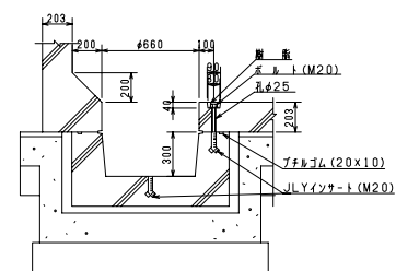
底設ピット S=1/20 断面図
