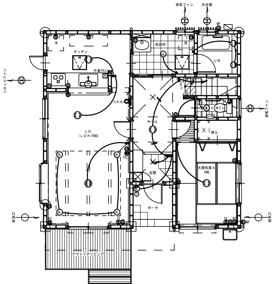
1階平面図 S=1/50
