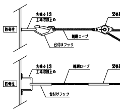
親綱ロープ取付詳細図
