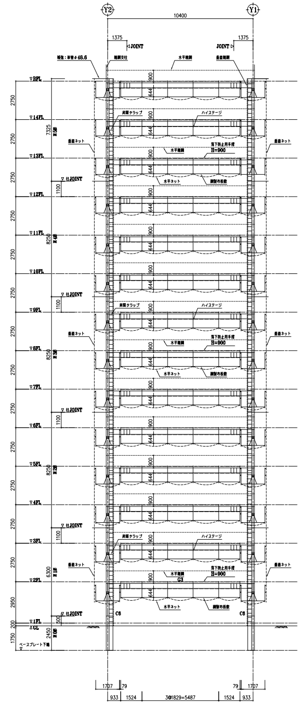
A-A断面図 S=1/100 (A3版 S=1/200)
