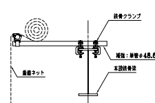
垂直養生ネット 取付詳細図 S=1/20 (A3版 S=1/40)
