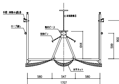
ハイステージ S・ピン式 S=1/20 (A3版 S=1/40)
