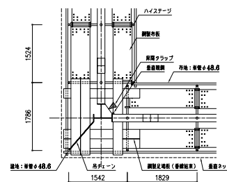
コナ一部平面詳細図 S=1/50 (A3版 S=1/100)
