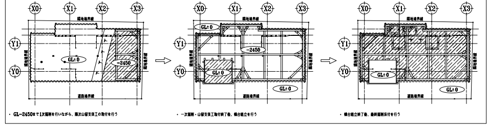
＜掘削順序フロー図＞
