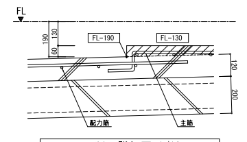
a-a断面詳細図 1/10
