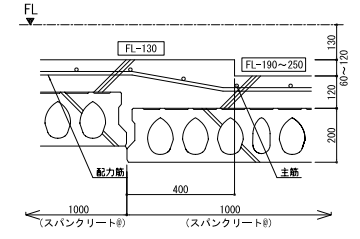
b-b断面詳細図 1/10
