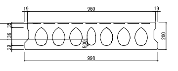
基準断面図 1/10
